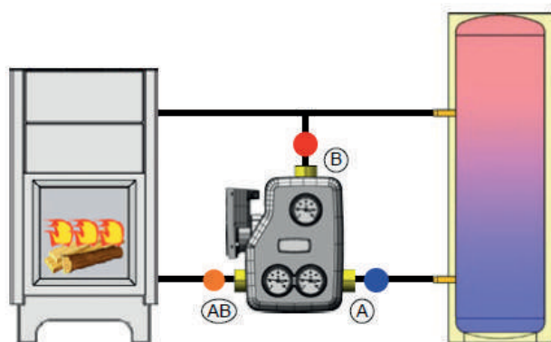
Schemă 1: Instalare pe dreapta
