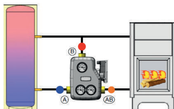
Schemă 1: Instalare pe stânga
