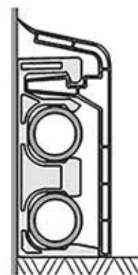
Secțiune transversală a conduței cu plintă
